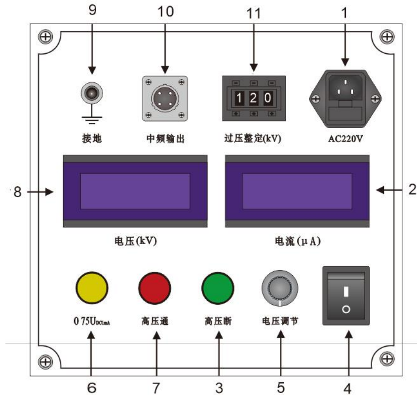
图2 面板布局图
