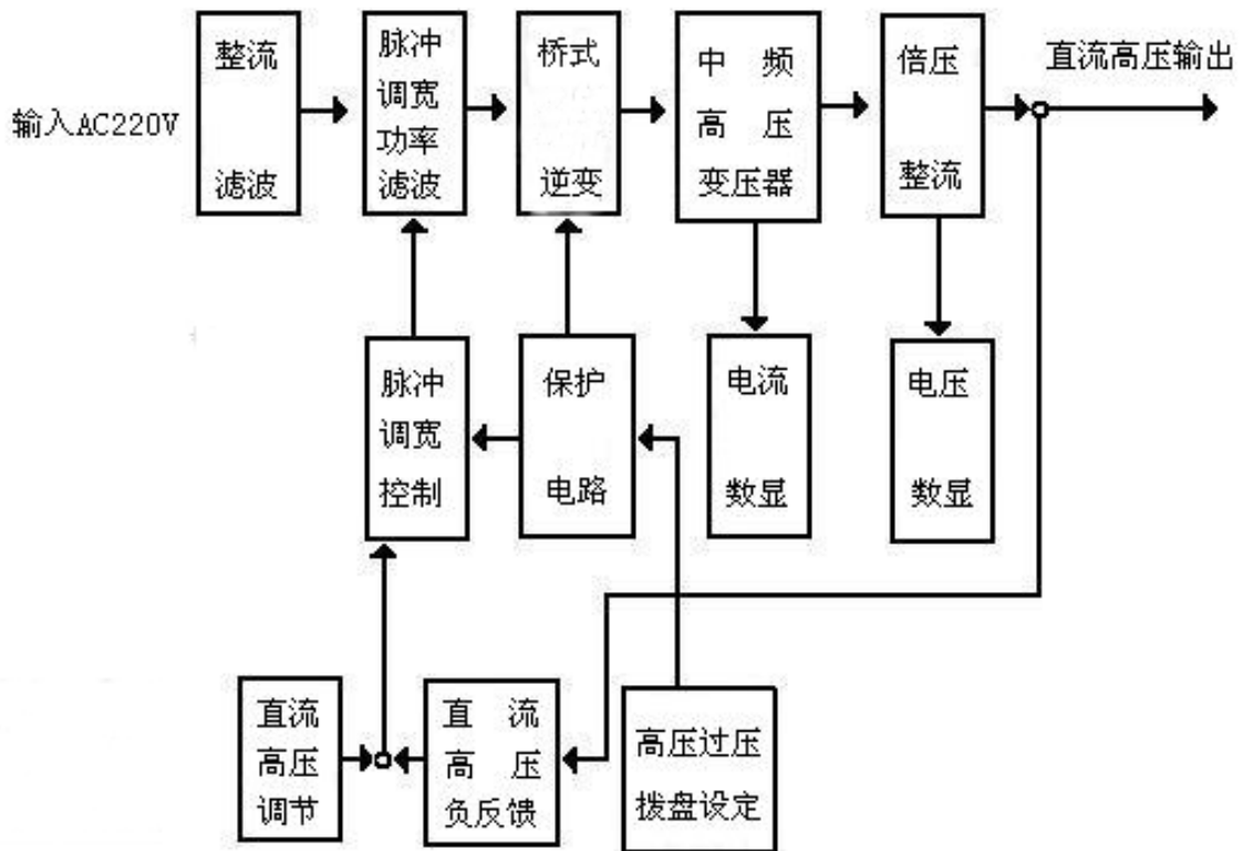
图 1 工作原理图
